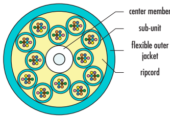
MTP® Mini Core Trunks
